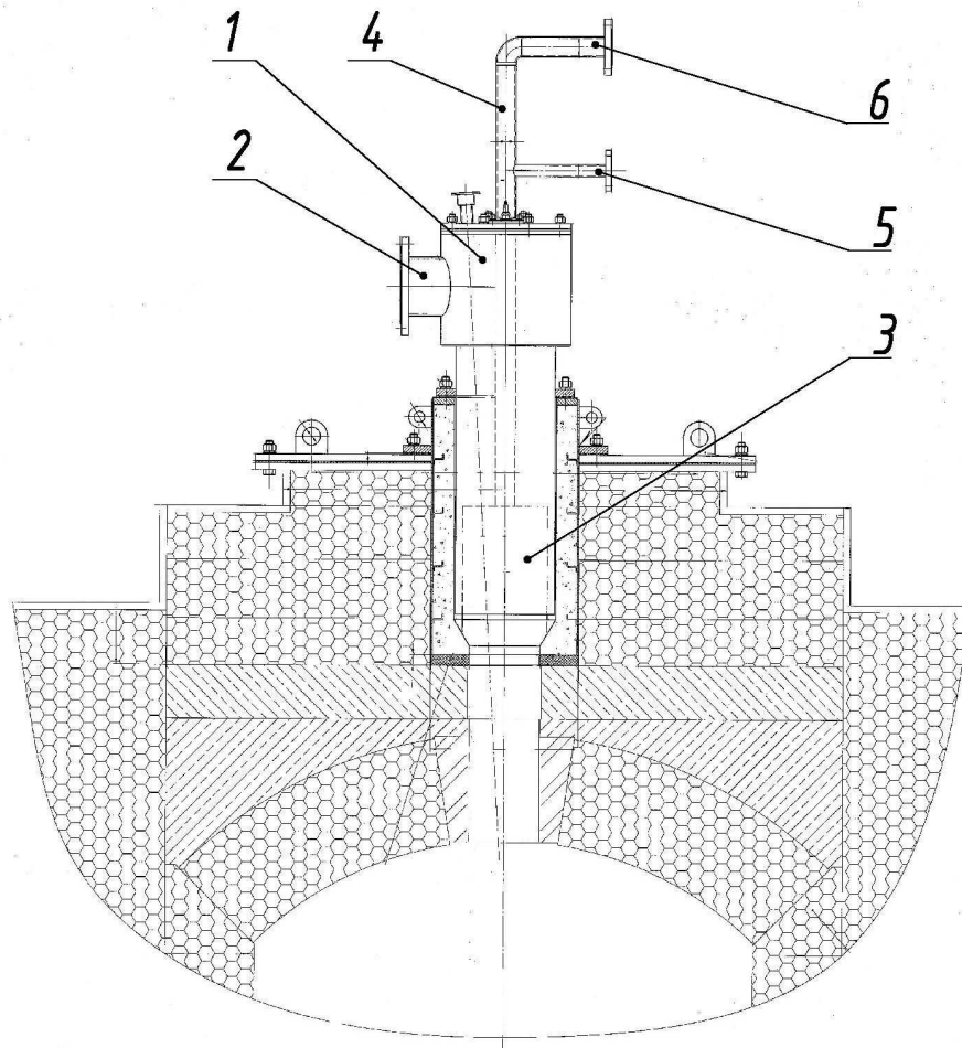
Рис. 3. Пусковая горелка
