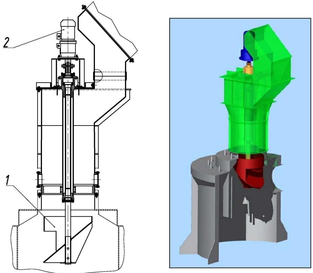
Рис. 2. Загрузочное устройство известняка
