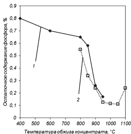
Рис. 3. Зависимость содержания фосфора в выщелоченном концентрате от температуры обжига: 1 – лабораторная вращающаяся печь; 2 – муфельная электропечь
