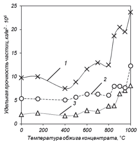
Рис. 2. Зависимость удельной прочности частиц концентрата от температуры прокаливания для различных фракций: 1 – фракция 0,315 – 0,160 мм, 2 – фракция 0,400 – 0,315 мм, 3 – фракция 0,630 – 0,400 мм
