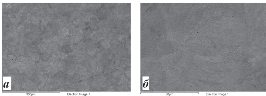
Рис. 10. Микроструктура верхней головки образца 0,57 % С после охлаждения в объеме масла: a – \times 200 ; б – \times 1000
