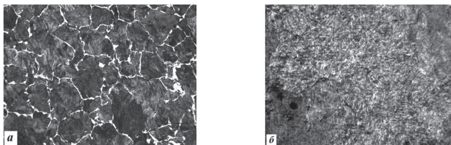
Рис. 7. Микроструктура нижней головки рельсовой накладки (0,53 %С) в горячекатаном состоянии (а) и после термоупрочнения в экспериментальном устройстве (б), \times 200
