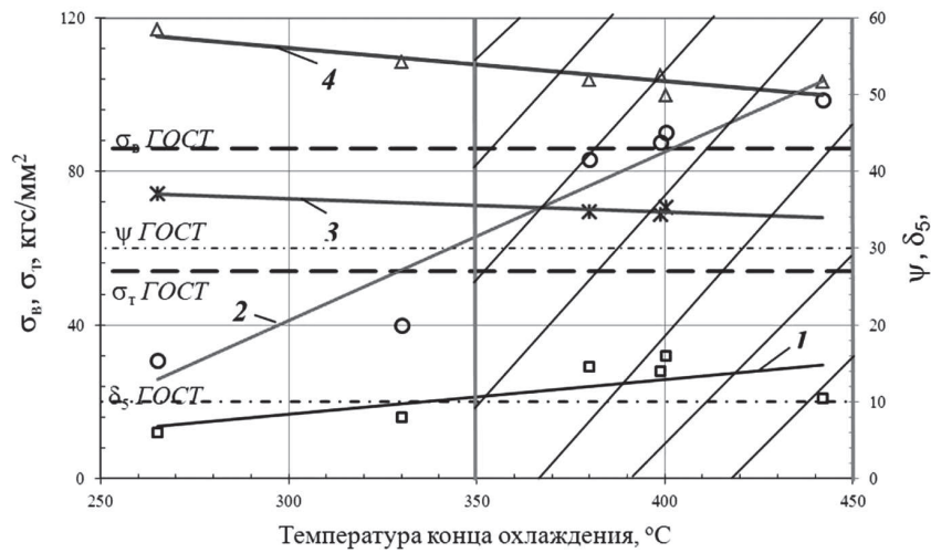
Рис. 5. Зависимость прочностных и пластических свойств рельсовой накладки Р65 от температуры конца охлаждения: 1 – относительное удлинение, 2 – относительное сужение, 3 – предел прочности, 4 – предел текучести
