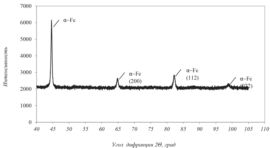
Рис. 9. Рентгенограмма середины шейки рельсовой накладки (0,53 %С)
