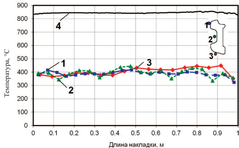
Рис. 4. Распределение температуры по длине накладки после выхода из устройства: 1, 2, 3 – температура поверхности по длине верхней головки, шейки и нижней головки соответственно; 4 – температура поверхности по длине шейки после выхода из печи до входа накладки в устройство охлаждения
