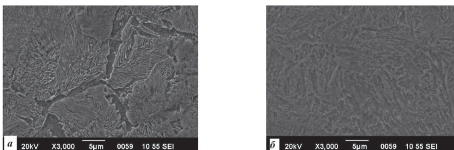
Рис. 8. Микроструктура середины верхней головки рельсовой накладки (0,53 %С) (а) и на расстоянии 500 мкм от кромки (б) после термоупрочнения в экспериментальном устройстве, \times 3000
