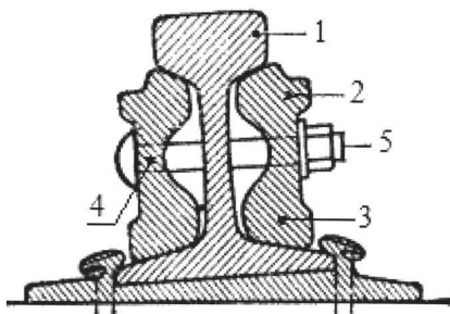
Рис. 1. Стандартный рельсовый стык с накладками Р65:
