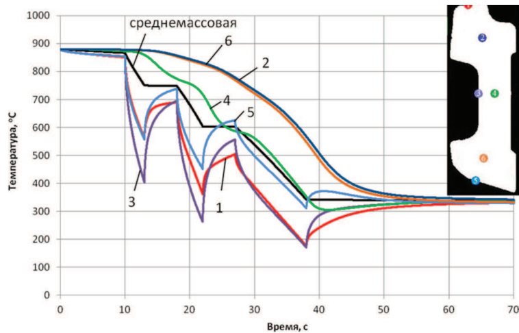
Рис. 2. Расчетное изменение температуры разных точек накладке во времени при двукратном прерывании охлаждения (номер и цвет кривой соответствует номеру и цвету расчетной точки)
