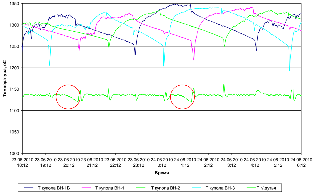
Рис. 9. Температуры купола и горячего дутья
