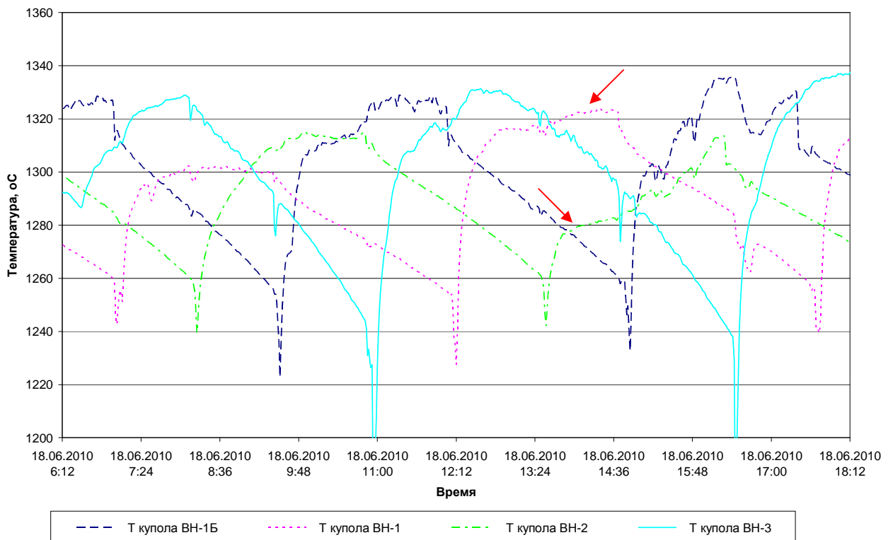
Рис. 4. Температура купола ВН
