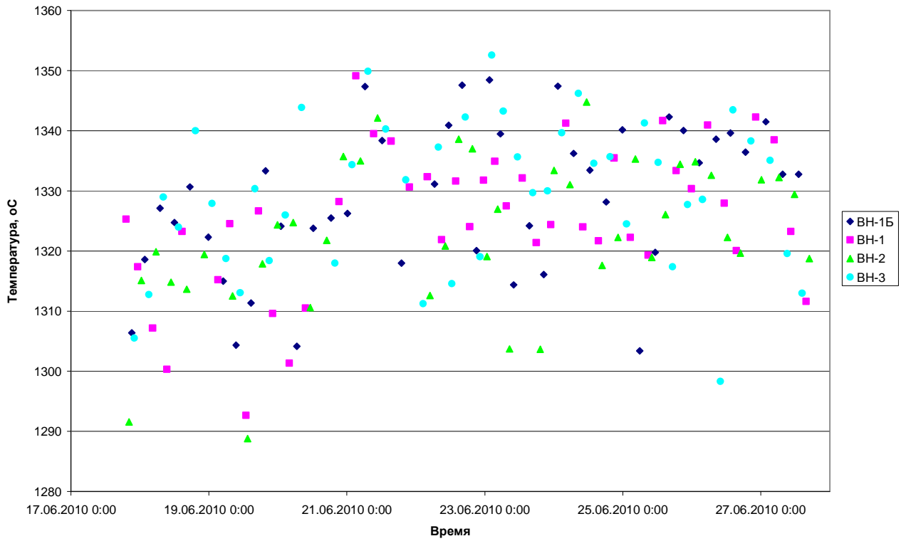
Рис. 3. Температура купола в конце газового периода
