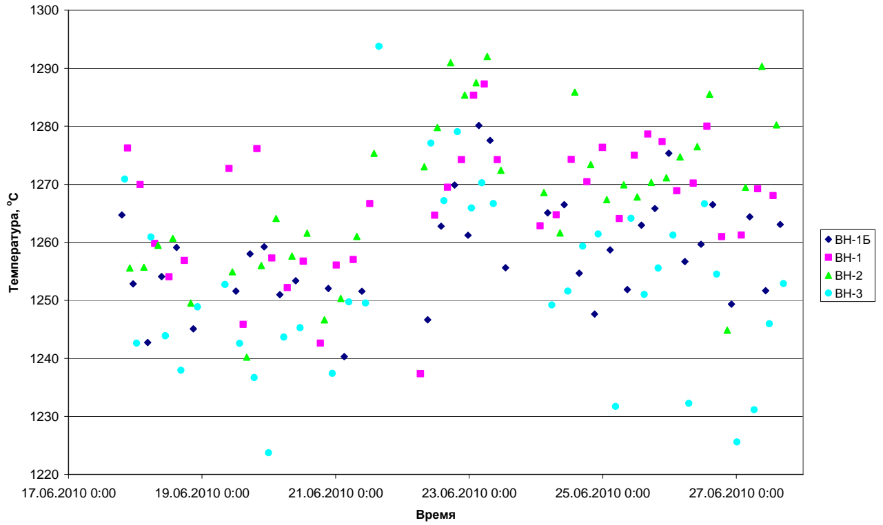
Рис. 7. Температура купола в конце дутьевого периода (минимальная)
